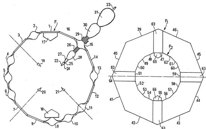
Рис. 130. Схема расположения электродов в устройстве Раватима.
