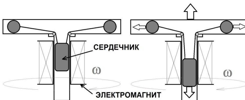
Рис. 31. Импульсный движитель Фролова.
