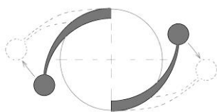
Рис. 126. Схема ротора с упругими элементами.
