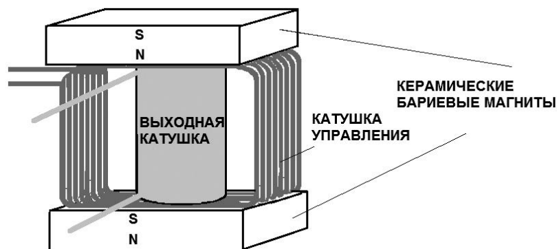
Рис. 59. Схема устройства Флойда Свита.
