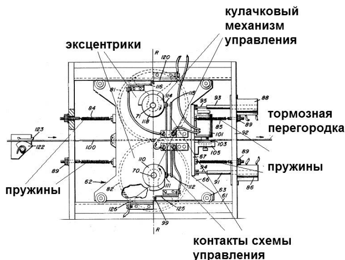
Рис. 36. Схема двигателя Нормана Дина.
