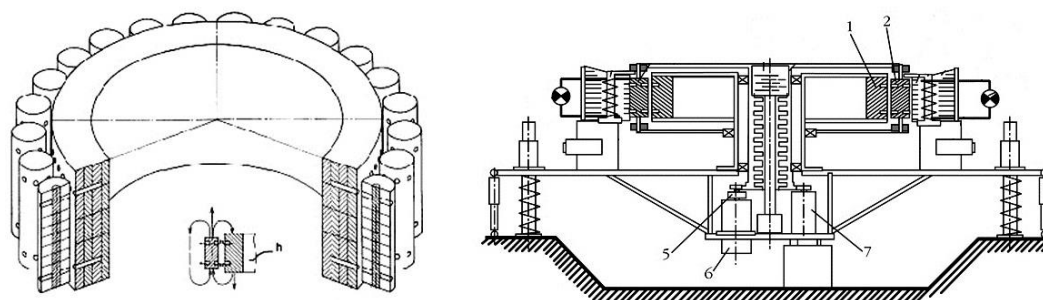
Рис.62. Установка «Астра», авторы Годин и Рощин, 1992 год.
