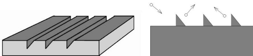
Рис.90 Варианты изготовления асимметричного микрорельефа
