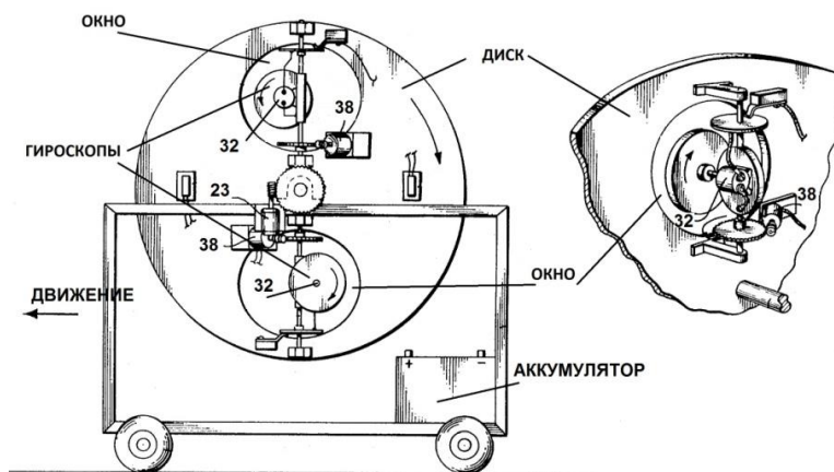
Рис. 49. Движитель с гироскопами, автор Ричард Фостер.
