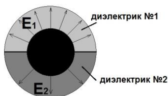
Рис. 85. Уединенное заряженное тело, окруженное разными диэлектриками.
