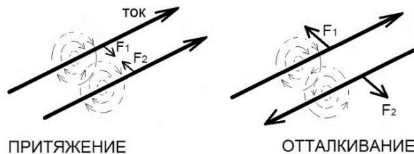
Рис. 12. Эффект Ампера для проводников с током.
