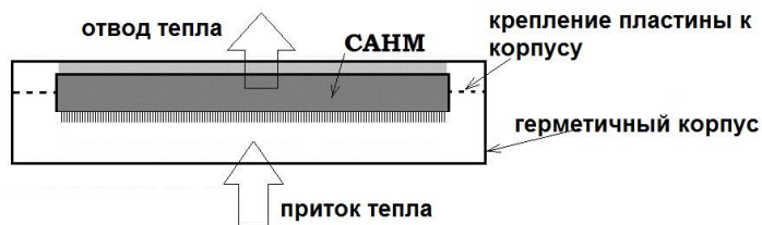
Рис. 96. САИМ в герметичном корпусе, заполненном газом.
