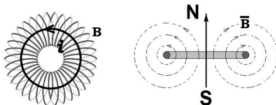
Рис. 53. Магнитное поле кольцевого тока.
