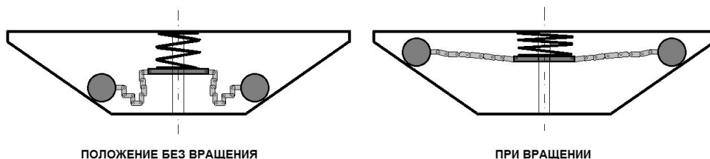
Рис. 32. Пара вращающихся грузиков на плоских цепях.
