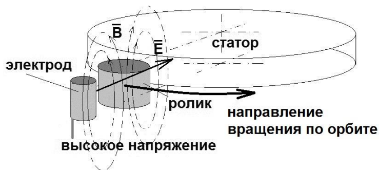
Рис. 63. Схема скрещенных электрических и магнитных полей.
