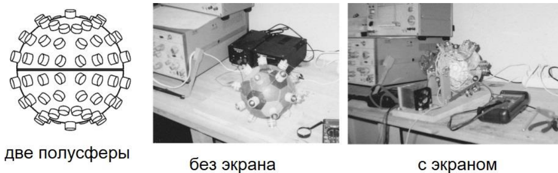
Рис. 157. Сферический корпус и излучатели в лаборатории Фролова, 2003 год.
