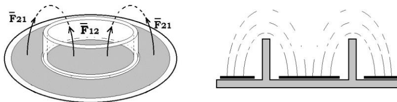
Рис. 78. Вариант конденсатора Фролова с цилиндрической перегородкой.
