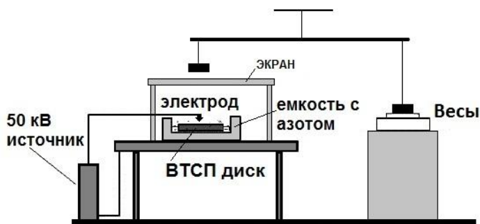
Рис.115. Схема эксперимента Фролова по влиянию электрического разряда на фазовое состояние охлажденного ВТСП материала.
