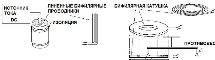
Рис. 110. Схема эксперимента Купера.
