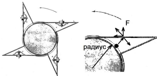
Рис. 104. Ротор заполнен газом или другой упругой средой.
