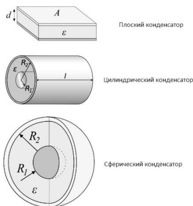
Рис. 128. Плоский, цилиндрический и сферический конженсаторы
