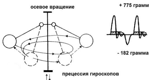
Рис.20. Силы, возникающие при прецессии гироскопов в эксперименте Полякова.
