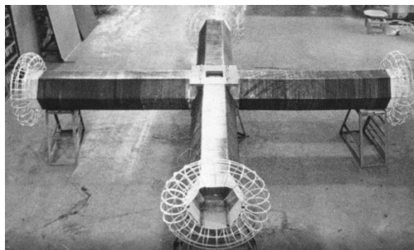
Рис. 68. Фотография пондеролета Игнатьева.
