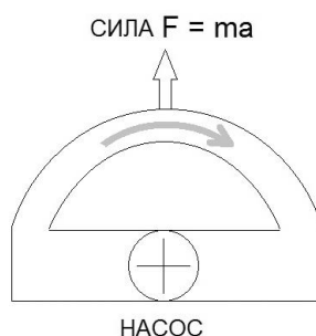
Рис. 17. Центробежная сила, возникающая при криволинейном движении жидкости по трубе.
