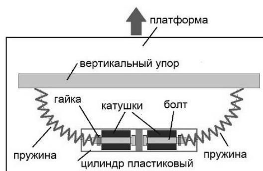
Рис. 45. Вариант движителя Фролова по схеме Шукалова
