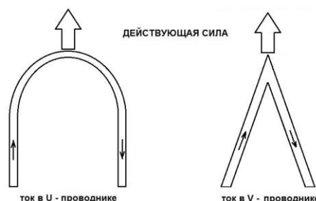
Рис.14. Эффект Сигалова в проводниках сложной формы.
