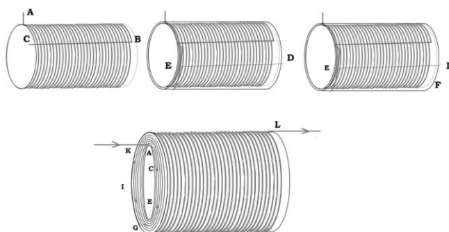
Рис.162. Многослойный соленоид.
