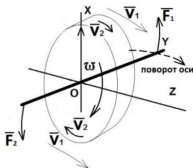
Рис. 47. Векторное сложение скоростей в верхней и нижней части гироскопа.
