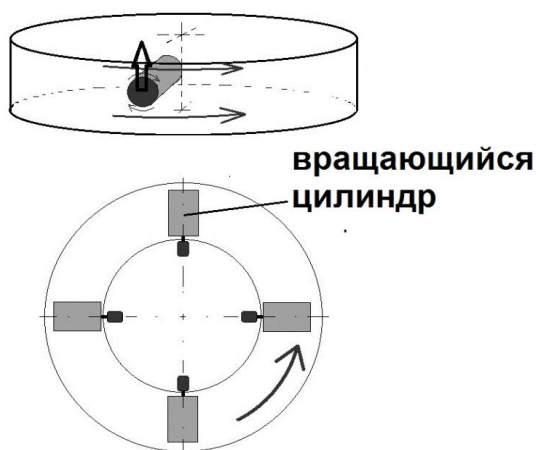
Рис.10. Двигатель на основе эффекта Магнуса.
