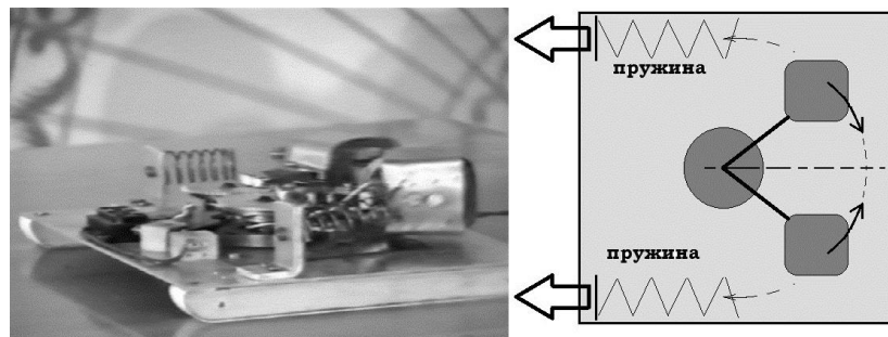
Рис. 44. Один из инерциоидов Шукалова.
