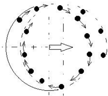
Рис. 48. Траектория точки на прецессирующем гироскопе.
