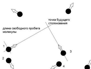
Рис. 88. Длина свободного пробега молекул газа.
