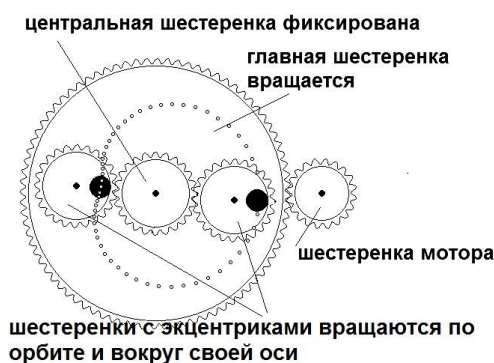
Рис. 42. Компьютерное моделирование инерциоиды Торнсона.
