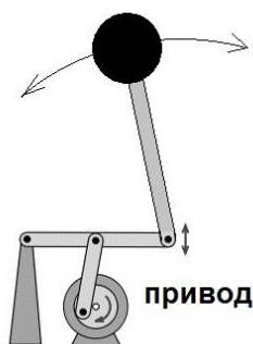
Рис. 28. Маятник Капицы.
