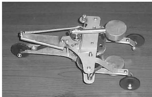
Рис. 33. Инерциод Толчина.
