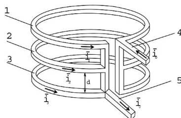
Рис. 156. Трехвитковый излучатель Черноброва.
