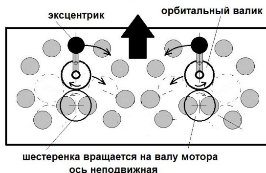
Рис. 41. Схема инерциоиды Торнсона.
