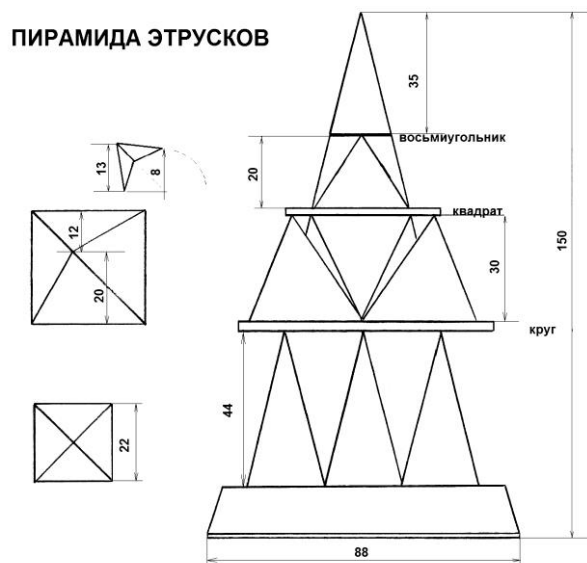
Рис.149. Схема пирамиды этрусков
