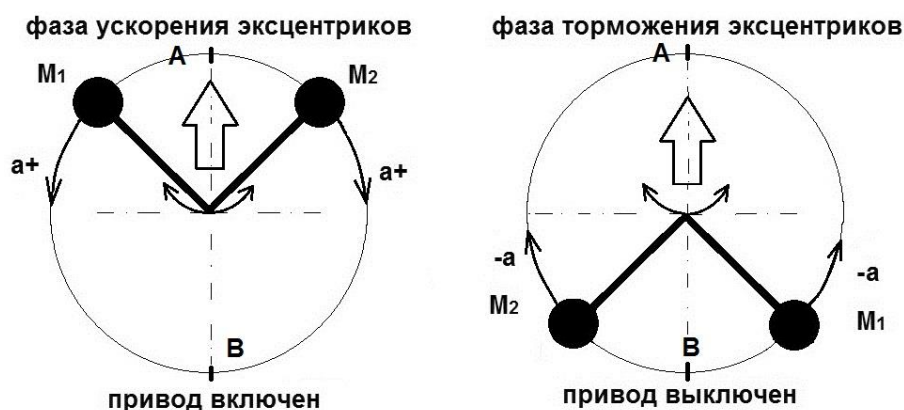
Рис. 34. Две фазы работы инерциода Толчина.
