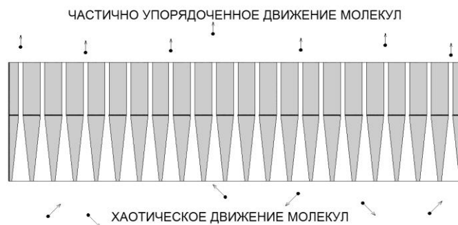
Рис. 94. Создание упорядоченного потока частиц газовой среды.
