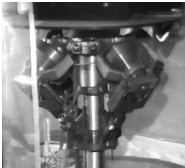
Рис. 18. Гироскопы движителя «Елка».
