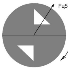
Рис. 108. Ротор с фрезеровкой полостей.
