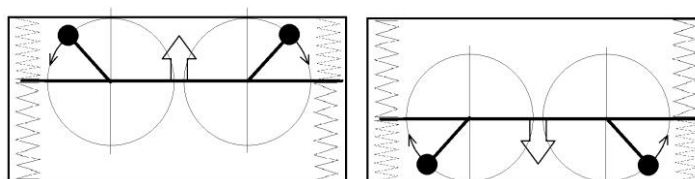
Рис. 37. Компенсация боковых колебаний двумя эксцентриками.
