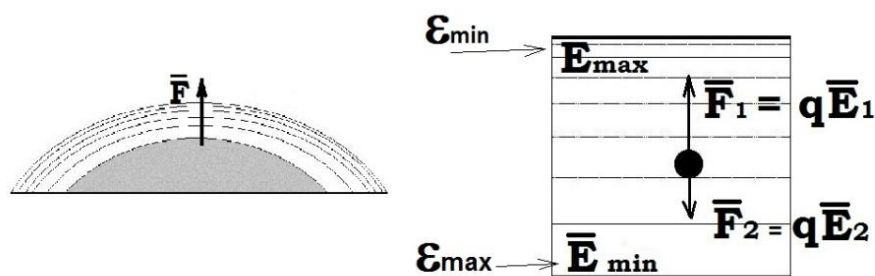
Рис. 83. Элемент активного движителя с градиентным диэлектриком.
