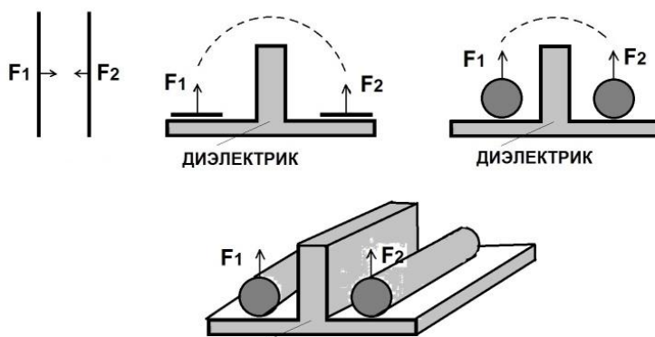
Рис. 77. Обычный конденсатор (слева) и конденсатор Фролова (справа)
