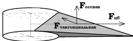
Рис. 107. Элемент ротора Фролова. Показаны осевая и тангенциальная составляющие силы.
