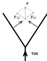
Рис.13. Силы в Y – образном проводнике электрического тока.
