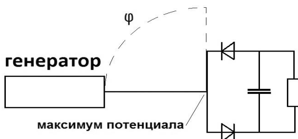
Рис.135. Однопроводная линия электропередач.
