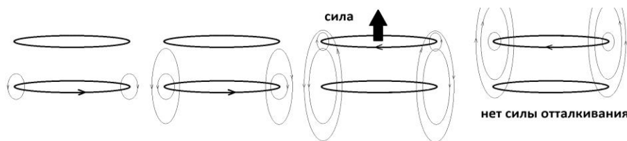
Рис.117. Два взаимодействующих импульсных электромагнита.
