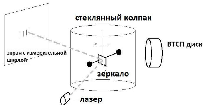
Рис. 114. Эксперимент с крутильными весами
