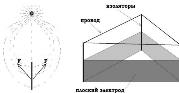
Рис. 74. Поле между двумя асимметричными электродами конденсатора.
