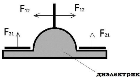
Рис. 76. Конденсатор Фролова, 1994 год. Асимметрия взаимодействия заряженных тел.
