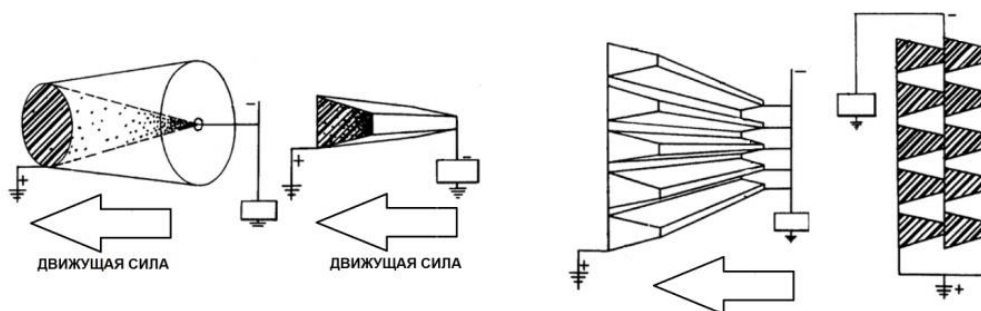
Рис. 73. Рисунки из патента Брауна.
