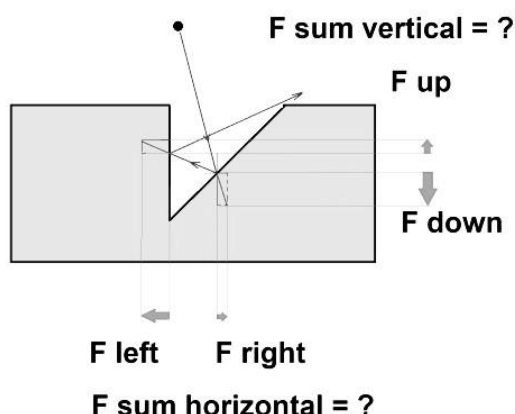
Рис.89 Вариант асимметричного микрорельефа и алгоритм расчет результирующего вектора сил
