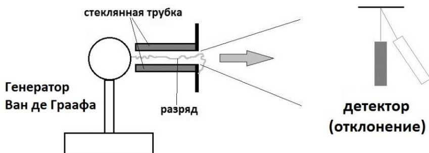
Рис. 113. Схема эксперимента Мортон.
