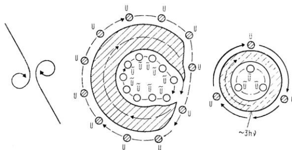
Рис. 119. Сжатие фотона и образование электрона, в модели Полякова.
