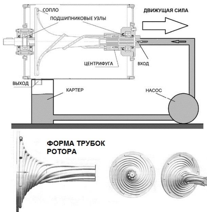
Рис. 4. Генератор Фролова по схеме Шаубергера.
