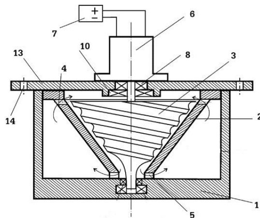
Рис. 23. Схема вихревого движителя Фролова.
