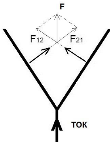
Рис.12. Силы в Y – образном проводнике электрического тока.
