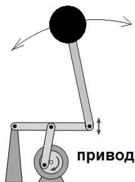
Рис. 27. Маятник Капицы.
