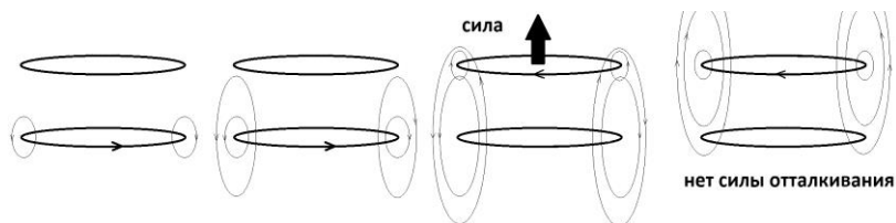
Рис.108. Два взаимодействующих импульсных электромагнита.
