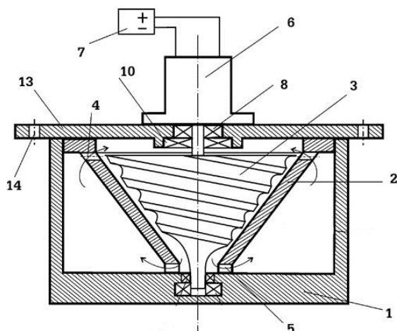
Рис. 22. Схема вихревого движителя Фролова.
