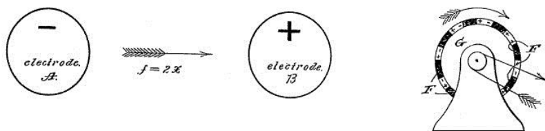
Рис. 68. Схема эффекта Брауна и его применение в роторе электрогенератора. Рисунки из патента.
