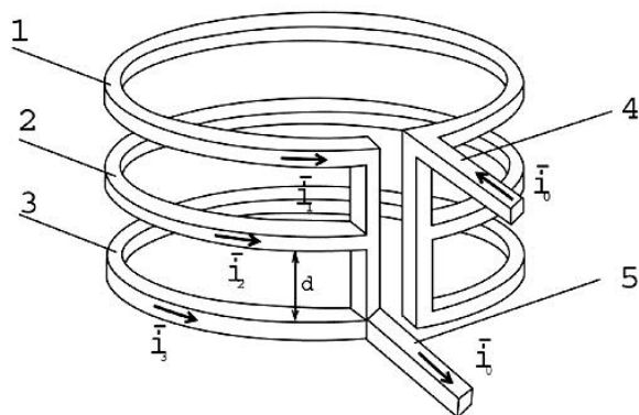
Рис. 144. Трехвитковый излучатель.
