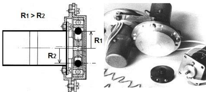
Рис.15. Движитель Вейника.
