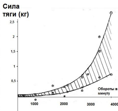
Рис.20. Вихревой двигатель Полякова и график зависимости силы тяги от оборотов.
