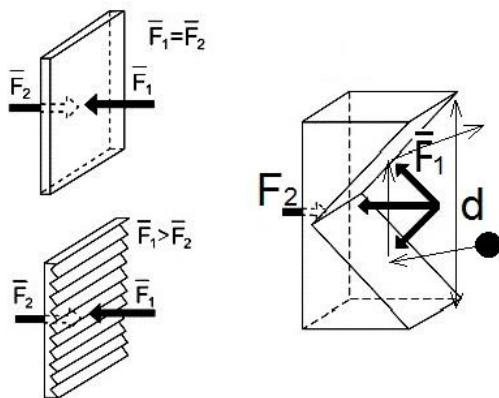
Рис. 82. Идея Михаила Порфирьевича Бешок по использованию энергии воздуха.
