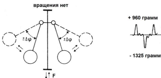
Рис.18. Калибровка устройства в эксперименте Полякова.
