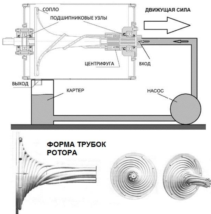
Рис. 4. Генератор Фролова по схеме Шаубергера.
