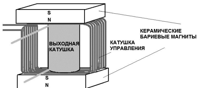
Рис. 56. Схема устройства Флойда Свита.
