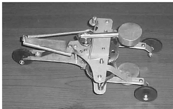
Рис. 31. Инерциоид Толчина.
