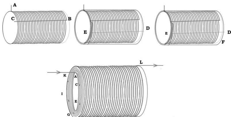
Рис.150. Многослойный соленоид.
