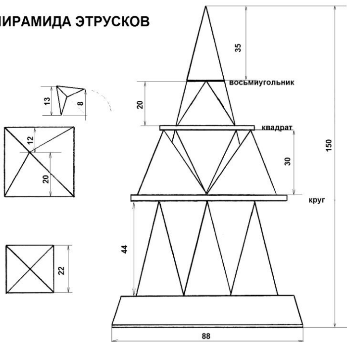
Рис.138. Схема пирамиды этрусков.
