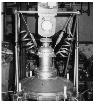
Рис.20. Вихревой двигатель Полякова и график зависимости силы тяги от оборотов.
