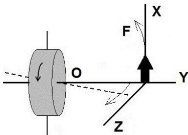
Рис. 43. Силы, возникающие при вынужденной прецессии оси гироскопа.
