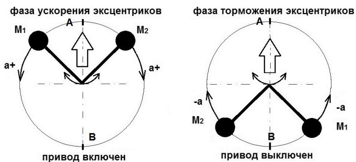
Рис. 32. Две фазы работы инерциоида.
