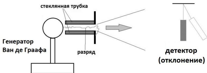
Рис. 104. Схема эксперимента Мортон.
