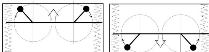
Рис. 35. Компенсация боковых колебаний двумя эксцентриками.
