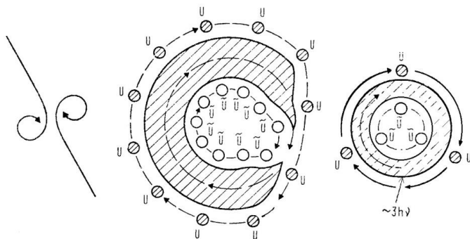
Рис. 110. Сжатие фотона и образование электрона, в модели Полякова.
