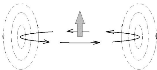
Рис. 102. Гравимагнитное поле вращающегося потока протонов (ионов водорода).
