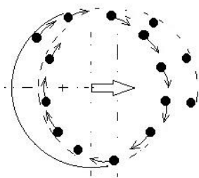
Рис. 45. Траектория точки на прецессирующем гироскопе.
