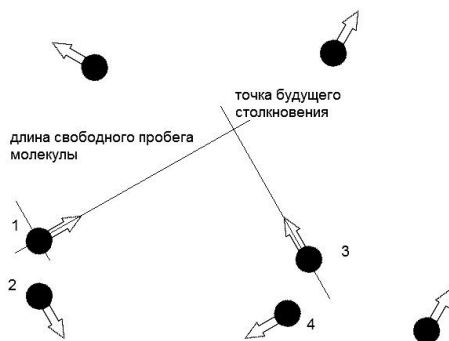
Рис. 83. Длина свободного пробега молекул газа.
