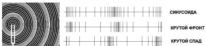
Рис. 118. Синусоидальная продольная волна, «толкающая» и «тянущая» волна.
