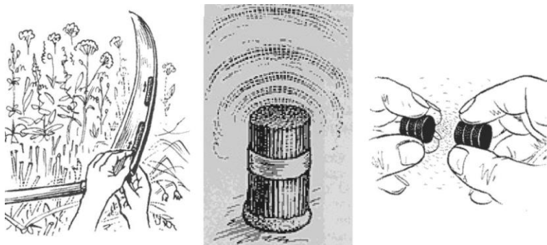
Рис. 128. Отталкивание двух стеблей или пучков травы.
