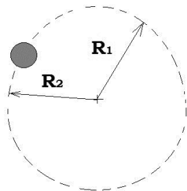
Рис. 53. Орбита электрона, имеющая эксцентриситет.
