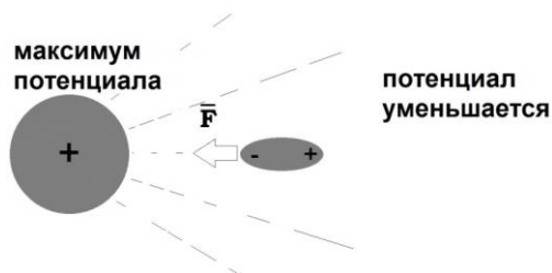
Рис. 78. Притяжение частицы к заряженному шарiku в естественном электрическом поле.
