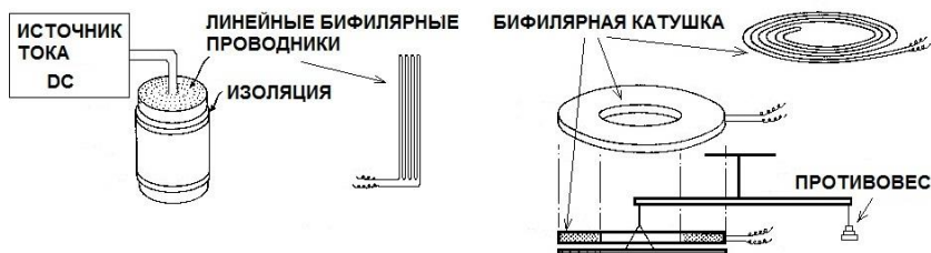
Рис. 101. Схема эксперимента Купера.
