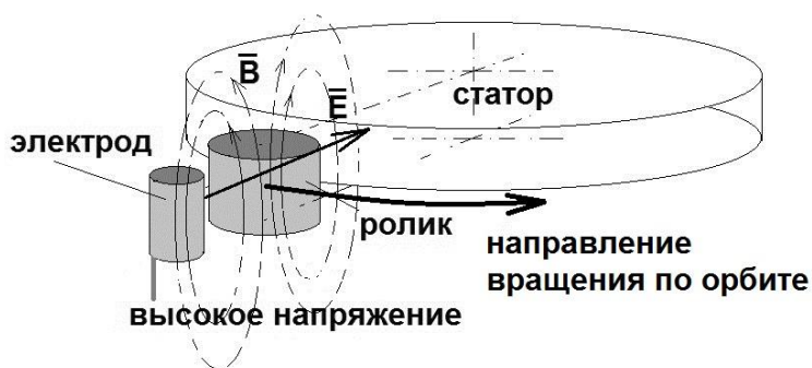
Рис. 60. Схема скрещенных электрических и магнитных полей.
