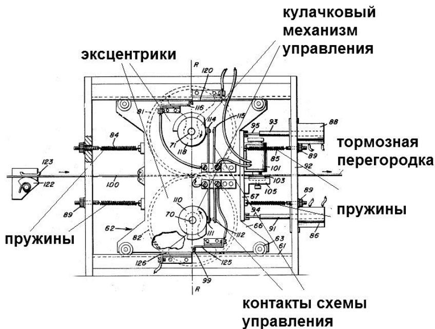
Рис. 34. Схема движителя Нормана Дина.
