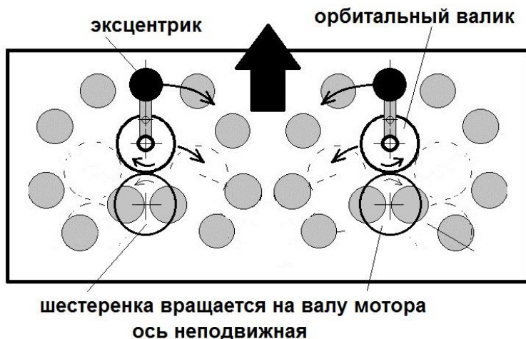
Рис. 39. Схема инерциоиды Торнсона.
