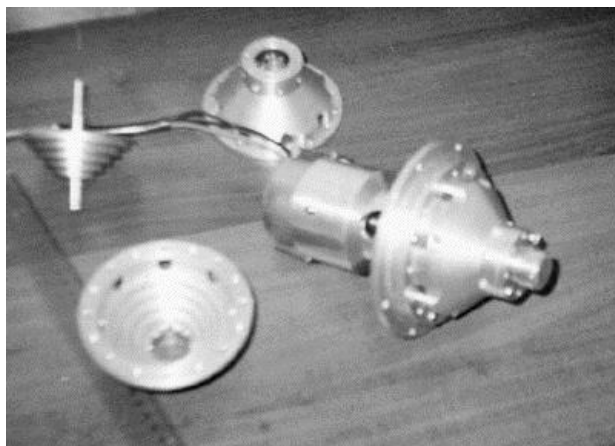
Рис. 23. Фото деталей экспериментального вихревого движителя, 2002 год.
