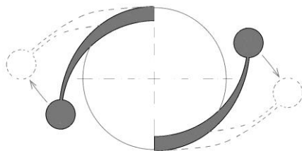
Рис. 117. Схема ротора с упругими элементами.
