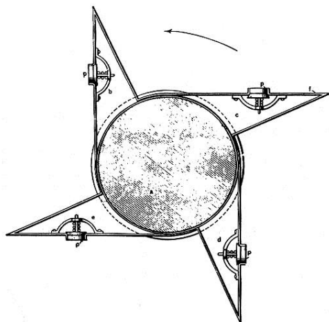
Рис. 95. Ротор заполнен газом или другой упругой средой.
