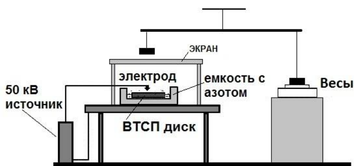
Рис.106. Схема эксперимента по влиянию электрического разряда на фазовое состояние охлажденного ВТСП материала.
