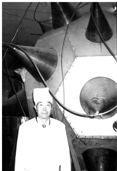
Рис. 121. Фотография одной из установок Цзяна.
