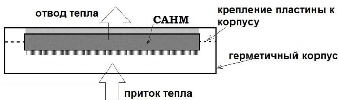
Рис. 89. САМ в герметичном корпусе, заполненном газом.
