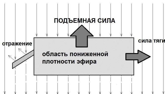
Рис. 55. Схема управления эфироплавательным аппаратом.
