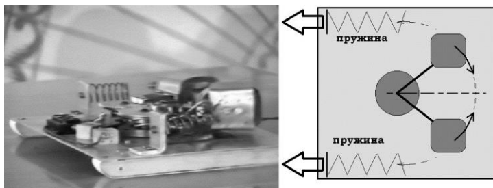
Рис. 42. Один из инерциодов Шукалова.
