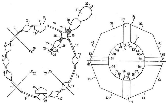
Рис. 120. Схема расположения электродов в устройстве Раватима.
