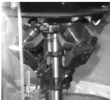
Рис. 17. Гироскопы движителя «Елка».
