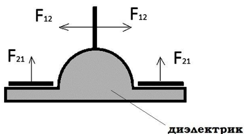
Рис. 72. Конденсатор Фролова, 1994 год. Асимметрия взаимодействия заряженных тел.
