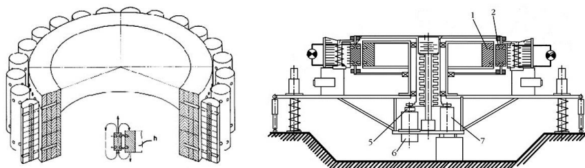
Рис.59. Установка «Астра», авторы Годин и Рощин, 1992 год.
