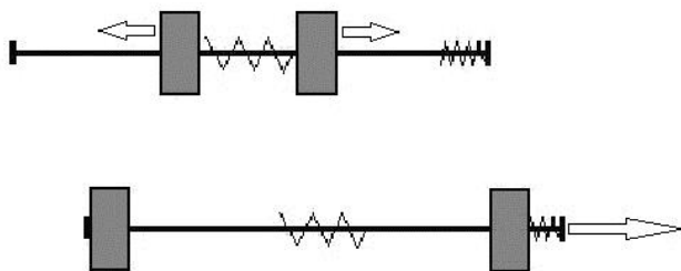
Рис.37. Эксперимент по упругому и неупругому взаимодействию.
