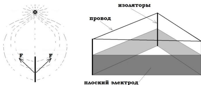
Рис. 70. Поле между двумя асимметричными электродами конденсатора.
