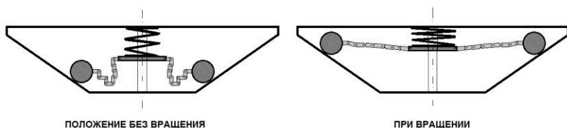
Рис. 30. Пара грузов на плоских цепях.
