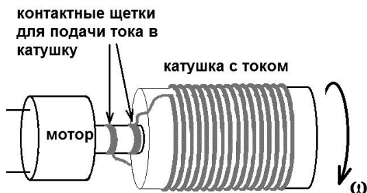
Рис. 103. Схема эксперимента с вращающимся контуром тока.
