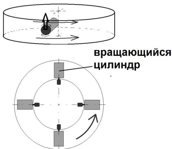
Рис.9. Двигатель на основе эффекта Магнуса.
