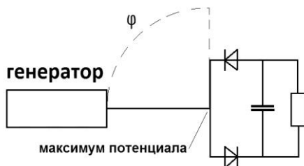
Рис.125. Однопроводная линия электропередач.
