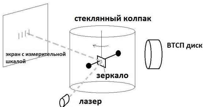
Рис. 105 Эксперимент с крутильными весами
