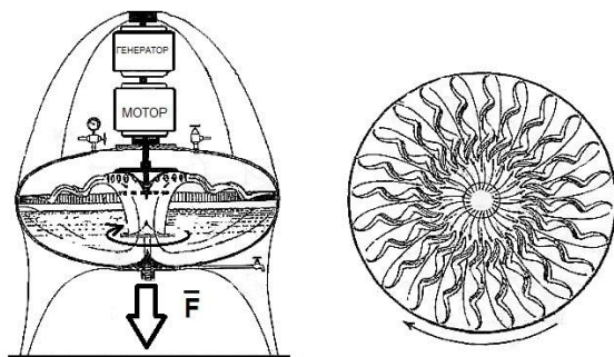
Рис.5 Генератор Шаубергера.
