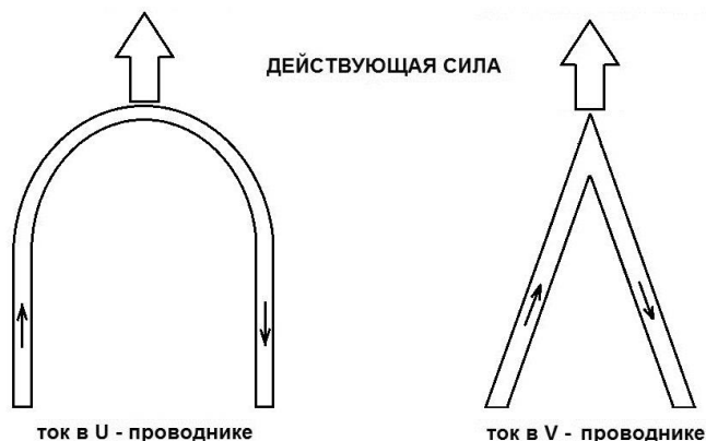
Рис.13. Эффект Сигалова в проводниках сложной формы.
