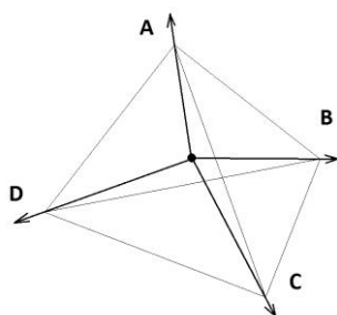
Рис. 142. Тетраэдрическая система координат.
