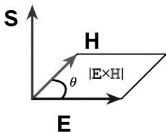
Рис. 62. Вектор Умова – Пойтинга S
