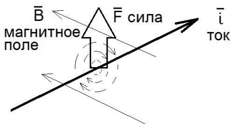
Рис.10. Сила Лоренца, как результат градиента давления эфира.
