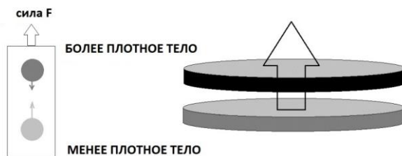
Рис. 93. Система двух гравитирующих тел разной плотности.
