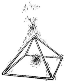
Рис. 137. Возникновение потоков эфира вблизи пирамиды.
