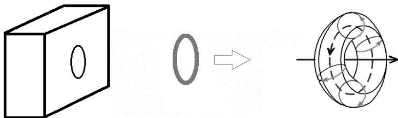
Рис. 111. Тороидальный вихрь и его движение.
