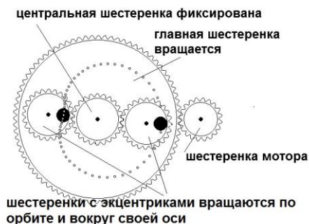
Рис. 40. Компьютерное моделирование инерциоида.
