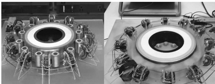
Рис. 57. Один из современных генераторов Серла.
