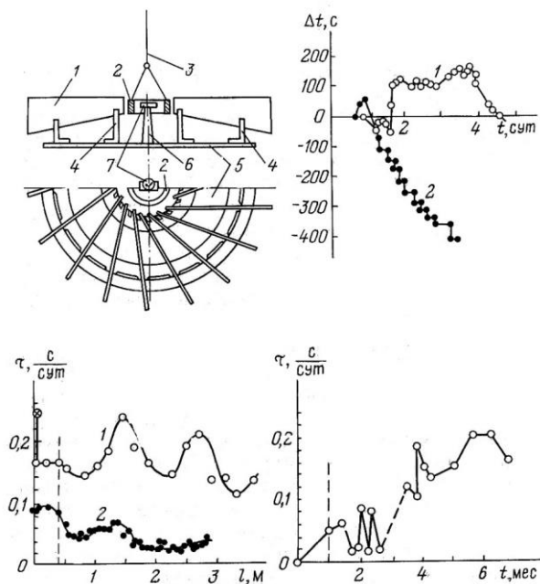
Рис. 123. Схема «касательного ежа» и графики измерений.
